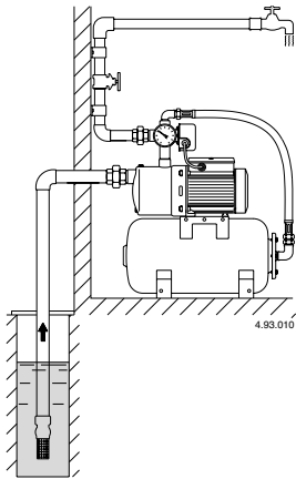
Fig. 2 Funzionamento in aspirazione Suction lift operation Saugbetrieb Fonctionnement en aspiration Funcionamiento en aspiración Sugande funktion Zuigsituatie Όψη λειτουργίας με κάθετη αναρρόφηση Работа в режиме всасывания
