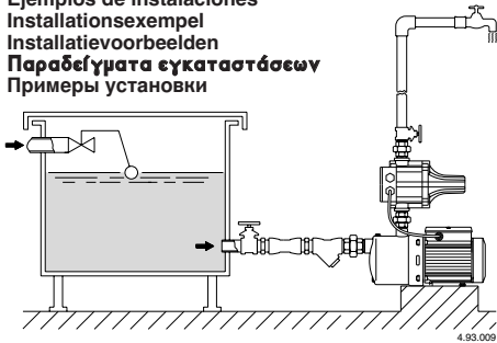
Fig. 1 Funzionamento sotto battente Positive suction head operation Zulaufbetrieb Fonctionnement en charge Funcionamiento bajo carga Tillrinning sugsidan Toeloopsituatie Όψη λειτουργίας με θετική αναρρόφηση Работа под гидравлическим напором
